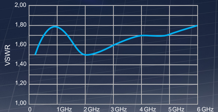
LP-04 - VSWR
